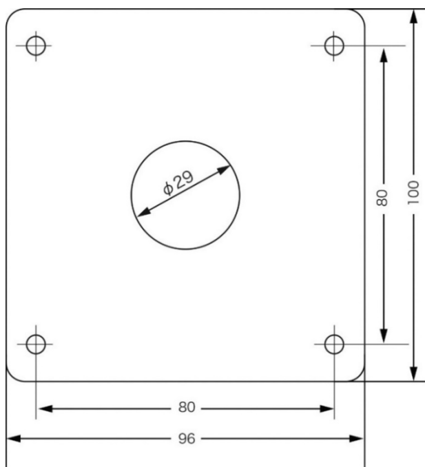
外形図
