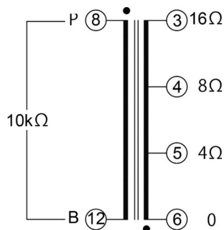
結線図
