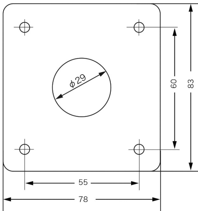
外形図
