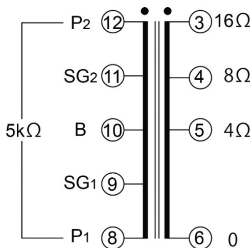
結線図
