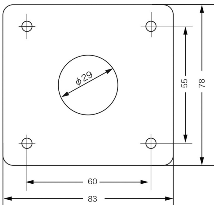
外形図
