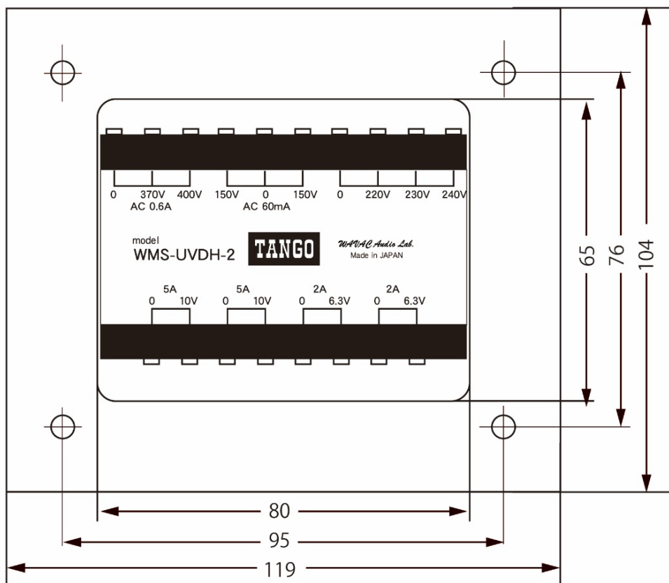
外形図
