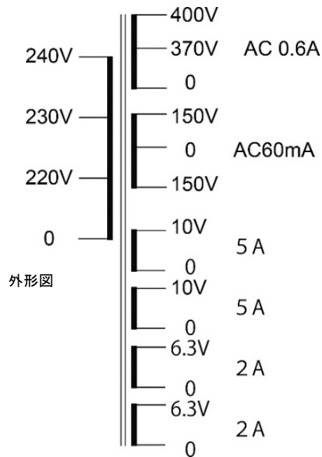
結線図
